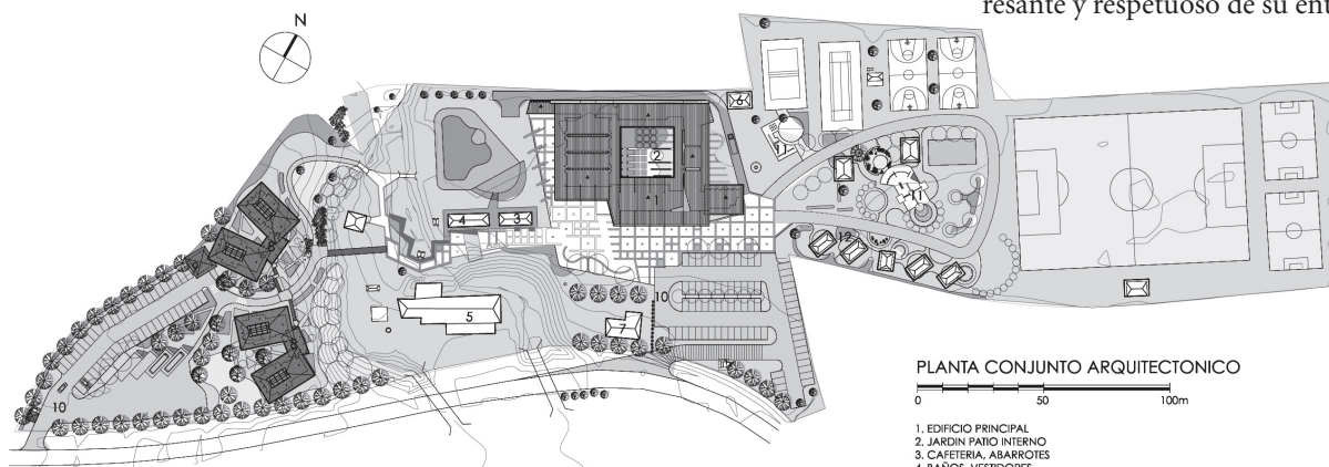
El diseño planteado para la construcción del nuevo Centro de Capacitación Integral Uxarraxi incluye cabañas, áreas verdes, espacio para el estudio y el esparcimiento, nuevos parqueos, restaurante y un edificio principal con salas de reuniones (imágenes del anteproyecto Sinergia).
